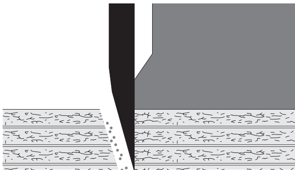
Schnittkante vor dem Messer Schnittkante hinter dem Messer
