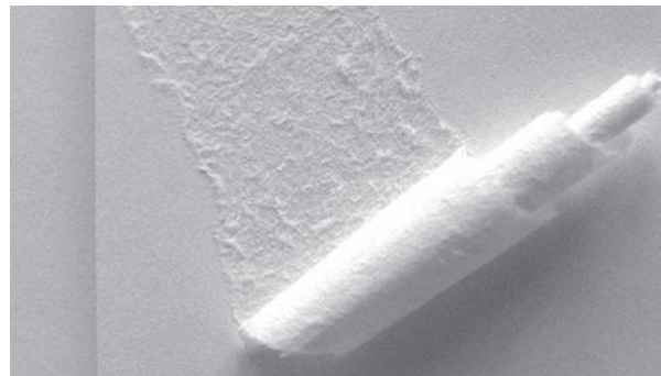
Ursprung eines Schälers an der Schnittkante (Schnittkante, vor dem Messer geschnitten – Schnittstaubpartikel oder unterster Bogen im Stapel).
